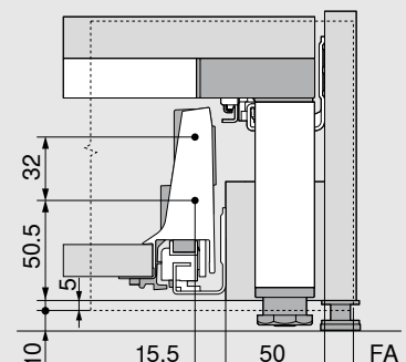
Konstrukční rozměry pro montáž čela vruty
