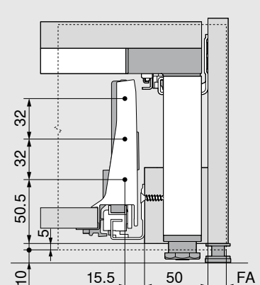
Konstrukční rozměry pro montáž čela vruty
